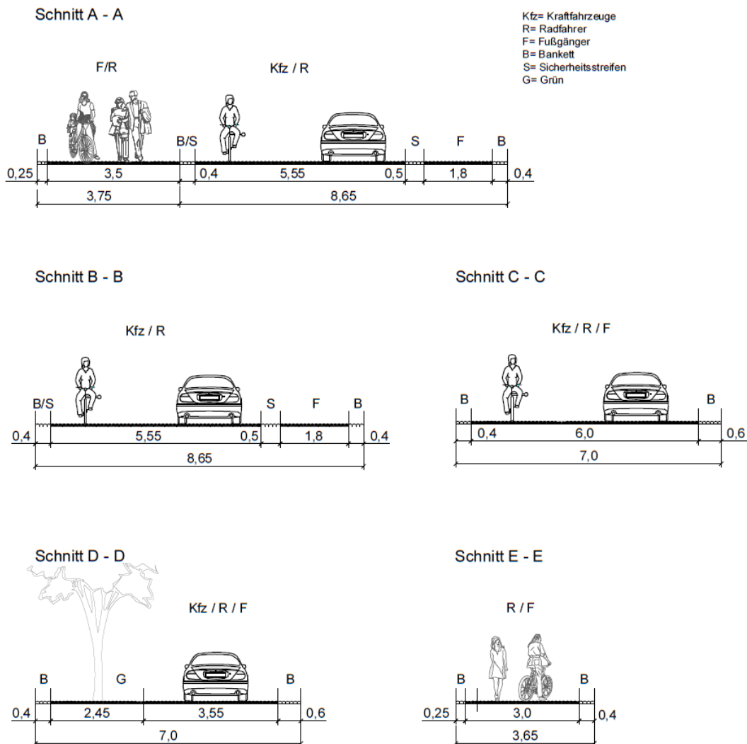
Abbildung 7: Empfohlene Straßenquerschnitte
